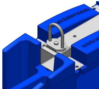
Fäste för bom 90x90
